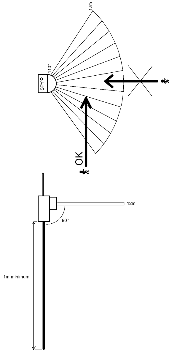
Montage détecteur SPY
